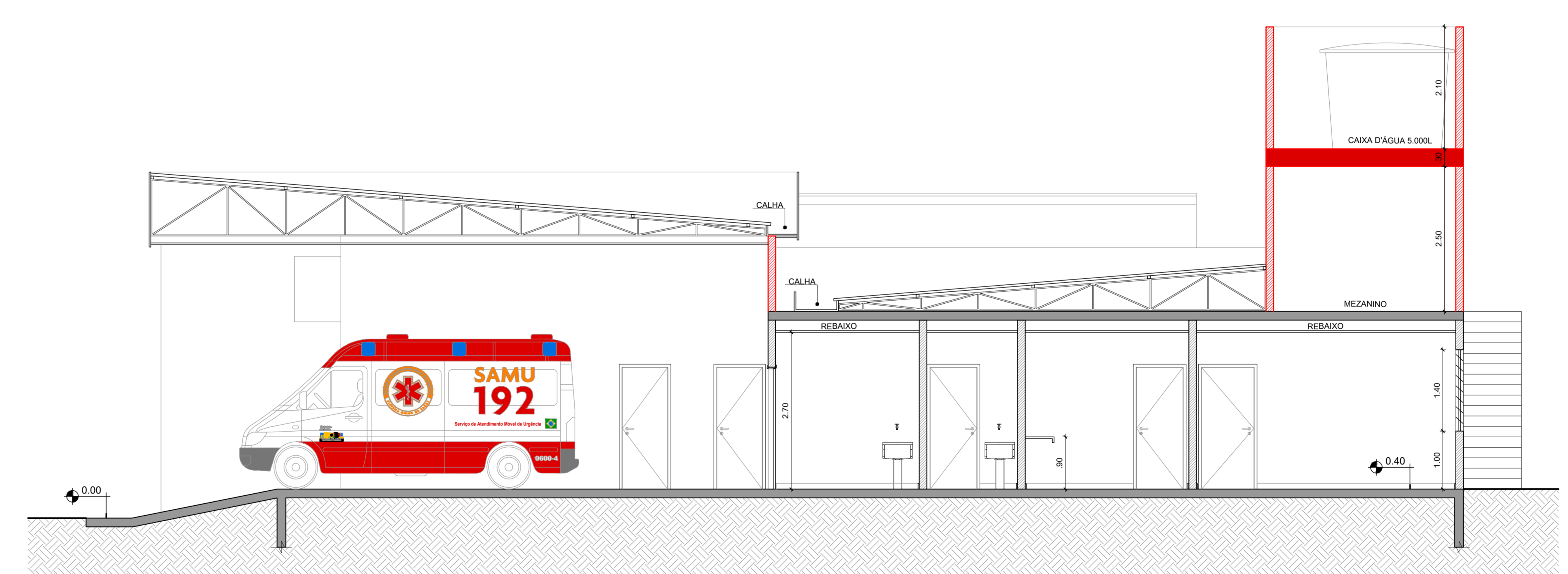
04 CORTE DD ESC. 1/50
