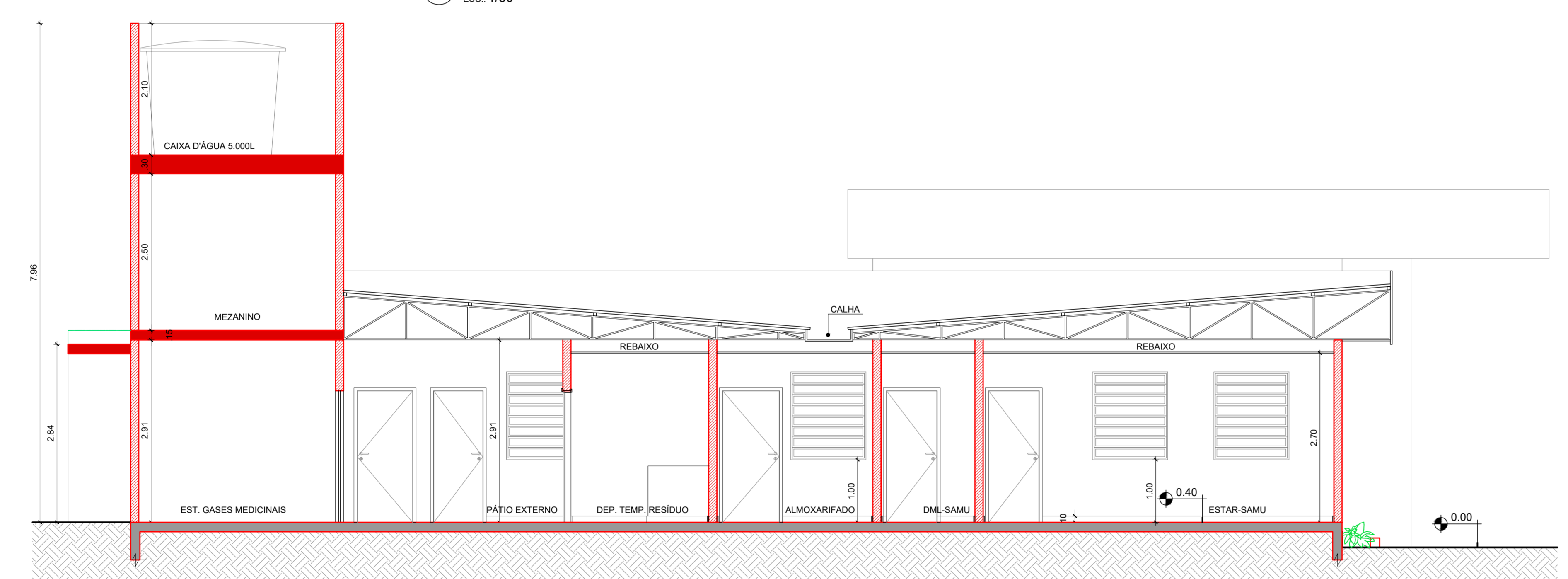
03 CORTE CC ESC. 1/50
