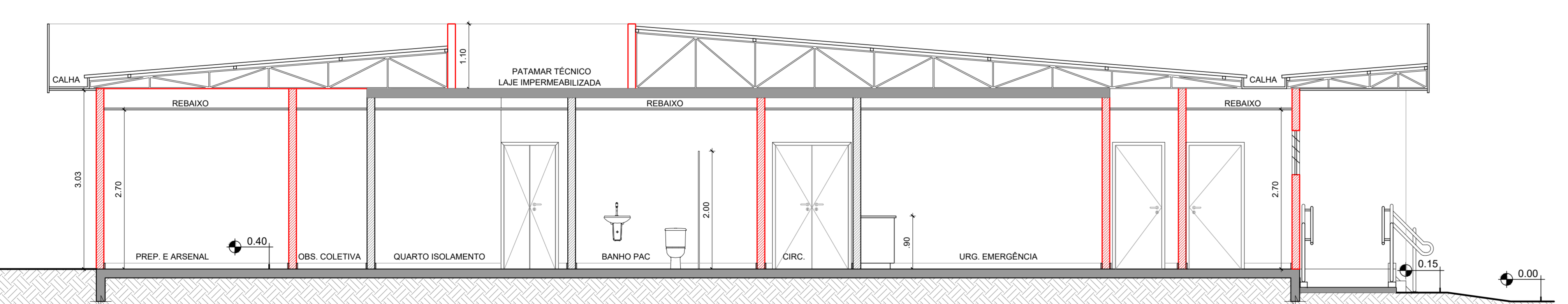
05 CORTE EE ESC. 1/50
